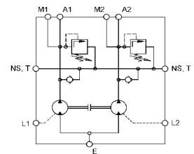
Sinnbild DIN ISO 1219
