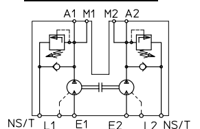
Sinnbild DIN ISO 1219
