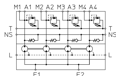
Sinnbild DIN ISO 1219
